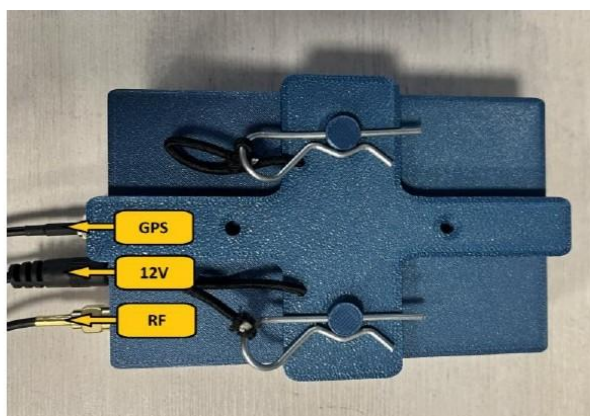
Soporte
